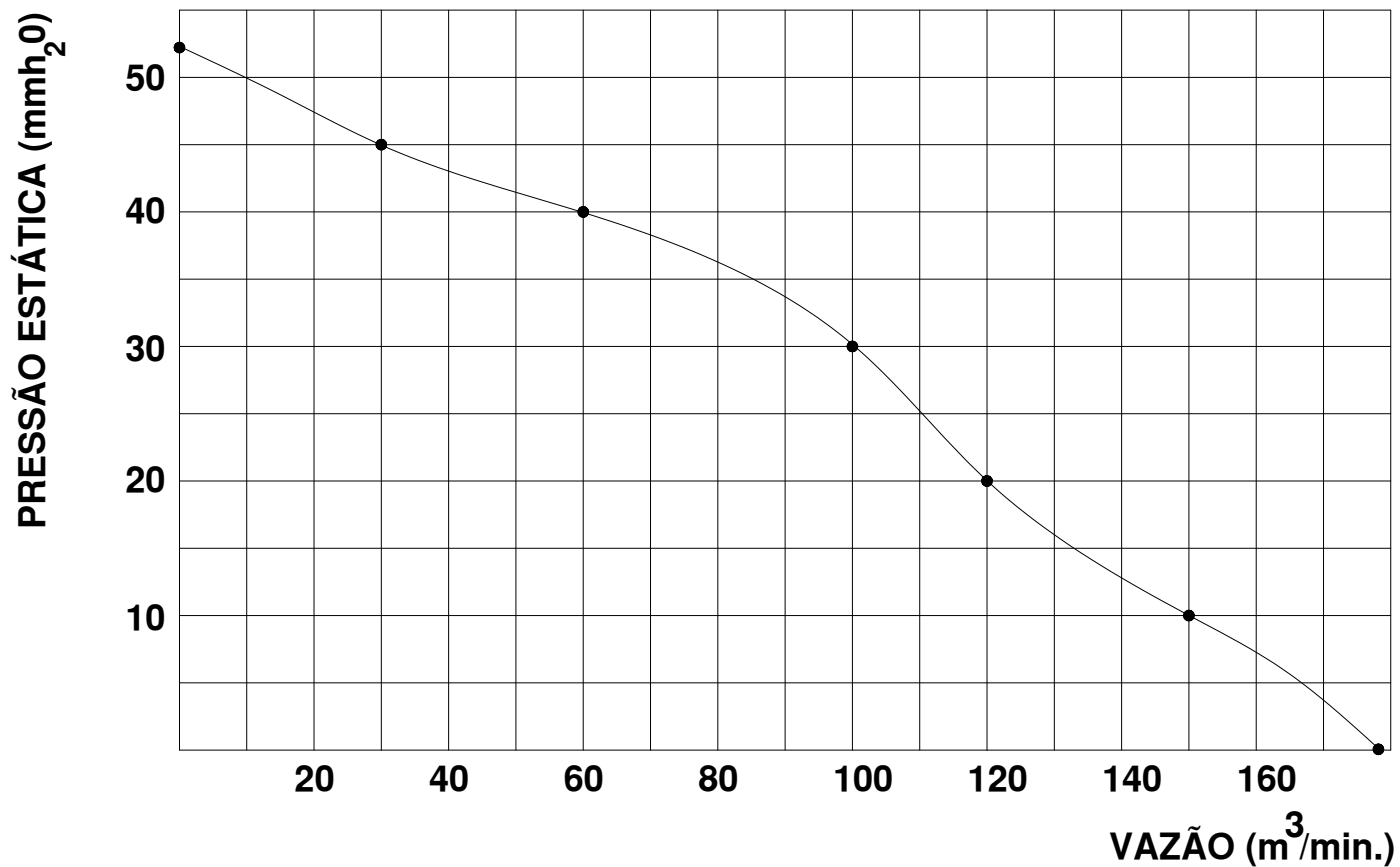
CURVA CARACTERÍSTICA ( 20^{\circ}\text{C}/760\text{ mm Hg} )
